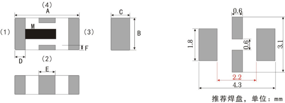
LFCN3216A系列产品外形结构图
