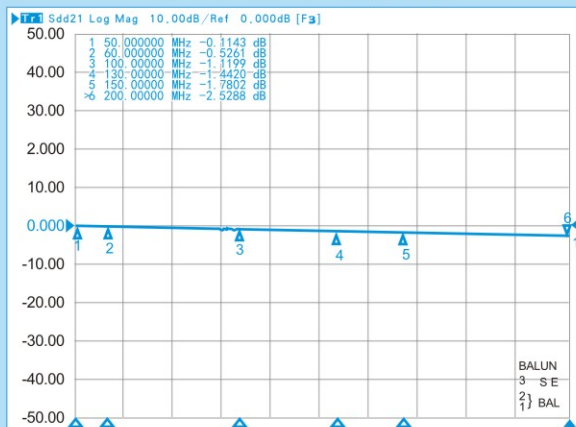
RFT4042A-1/4 插入损耗
