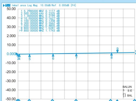
RFT4042A-4/1 幅度不平衡
