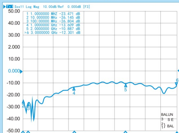
RFT4042G-1/1 返回损耗
