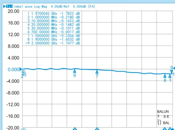
RFT4042H-4/1 幅度不平衡
