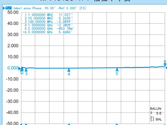
RFT4042G-1/1 相位不平衡
