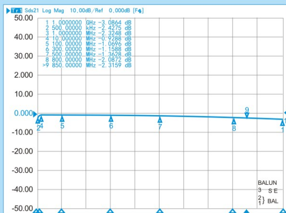
RFT4042A-4/1 插入损耗
