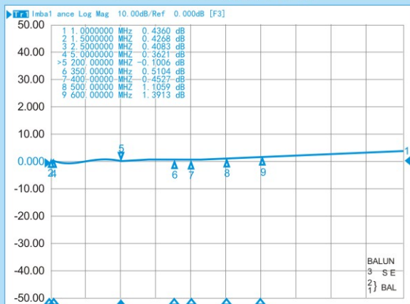
RFT4042C-1/1 幅度不平衡
