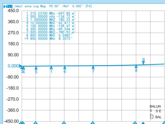
RFT4042A-4/1 相位不平衡
