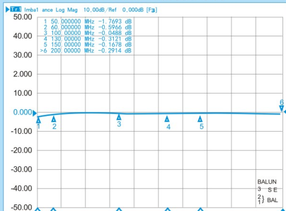
RFT4042A-1/4 幅度不平衡
