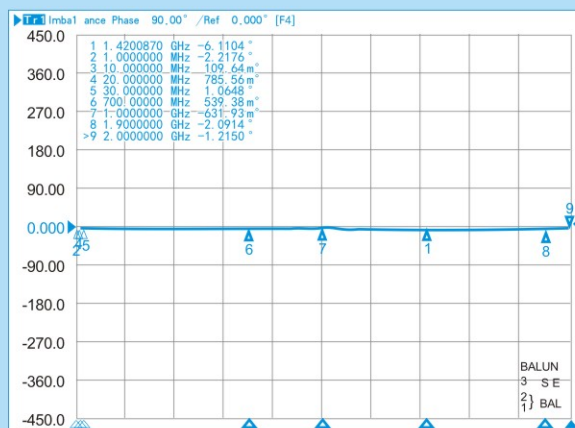
RFT4042H-4/1 相位不平衡
