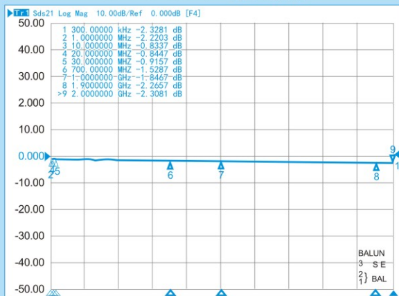
RFT4042H-4/1 插入损耗
