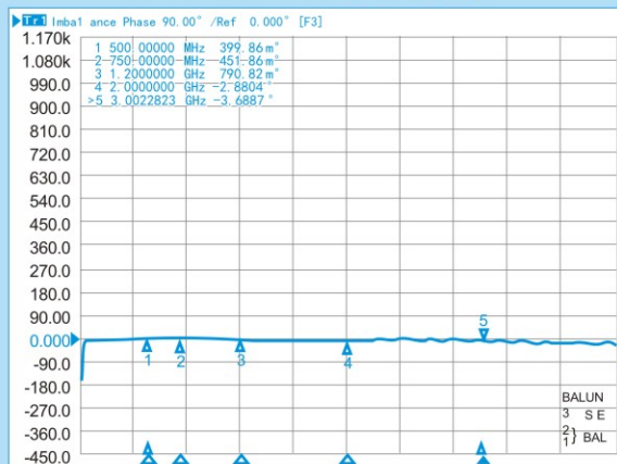
RFT4042H-4/1A 相位不平衡
