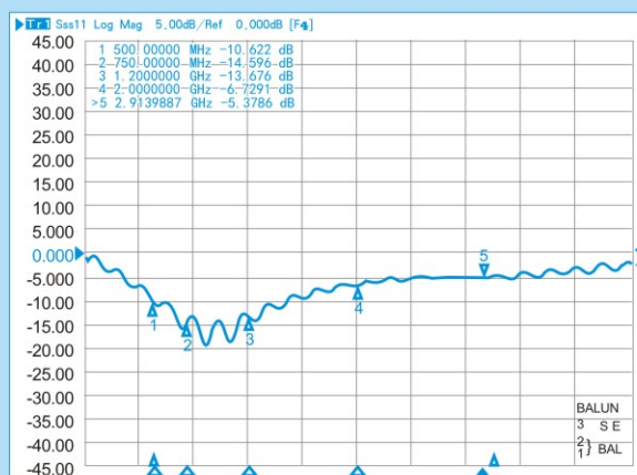
RFT4042H-4/1A 返回损耗
