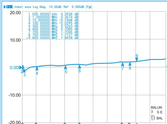
RFT4042A-1/1 幅度不平衡
