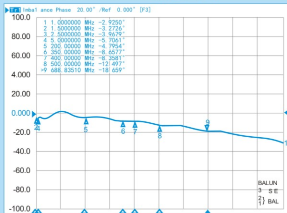
RFT4042C-1/1 相位不平衡
