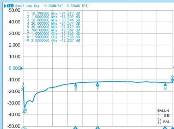
RFT4042H-4/1 返回损耗
