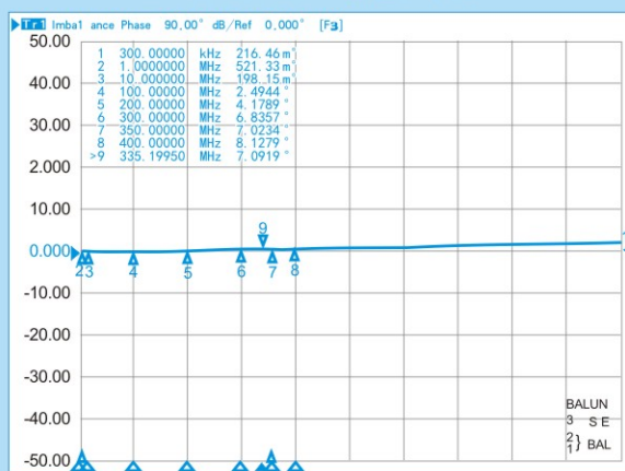
RFT4042A-2/1 相位不平衡
