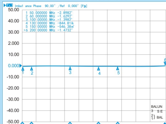
RFT4042A-1/4 相位不平衡
