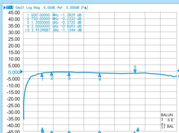
RFT4042H-4/1A 插入损耗
