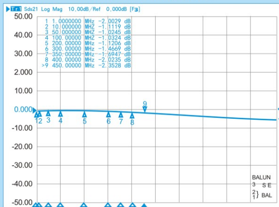
RFT4042A-2/1 插入损耗
