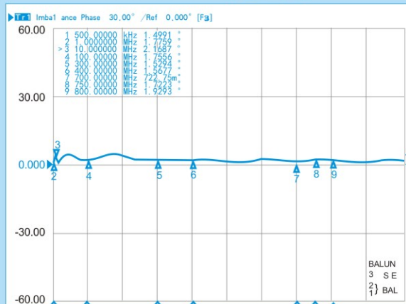
RFT4042A-1/1 相位不平衡
