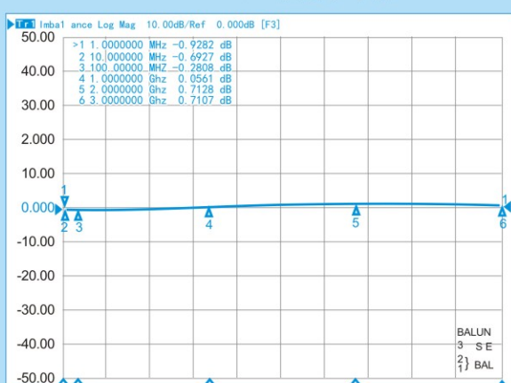
RFT4042G-1/1 幅度不平衡
