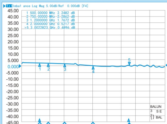
RFT4042H-4/1A 幅度不平衡
