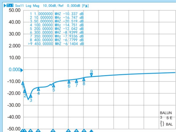
RFT4042A-2/1 返回损耗
