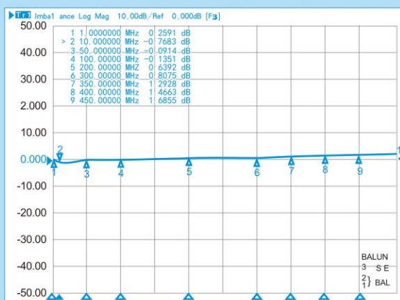
RFT4042A-2/1 幅度不平衡
