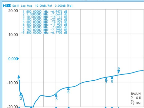
RFT4042A-1/1 返回损耗
