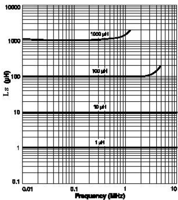
Ls vs Frequency 特性曲线
