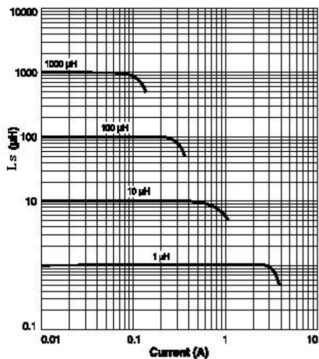
Ls vs Current 特性曲线
